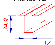
EMENDA PERFIL PRINCIPAL
